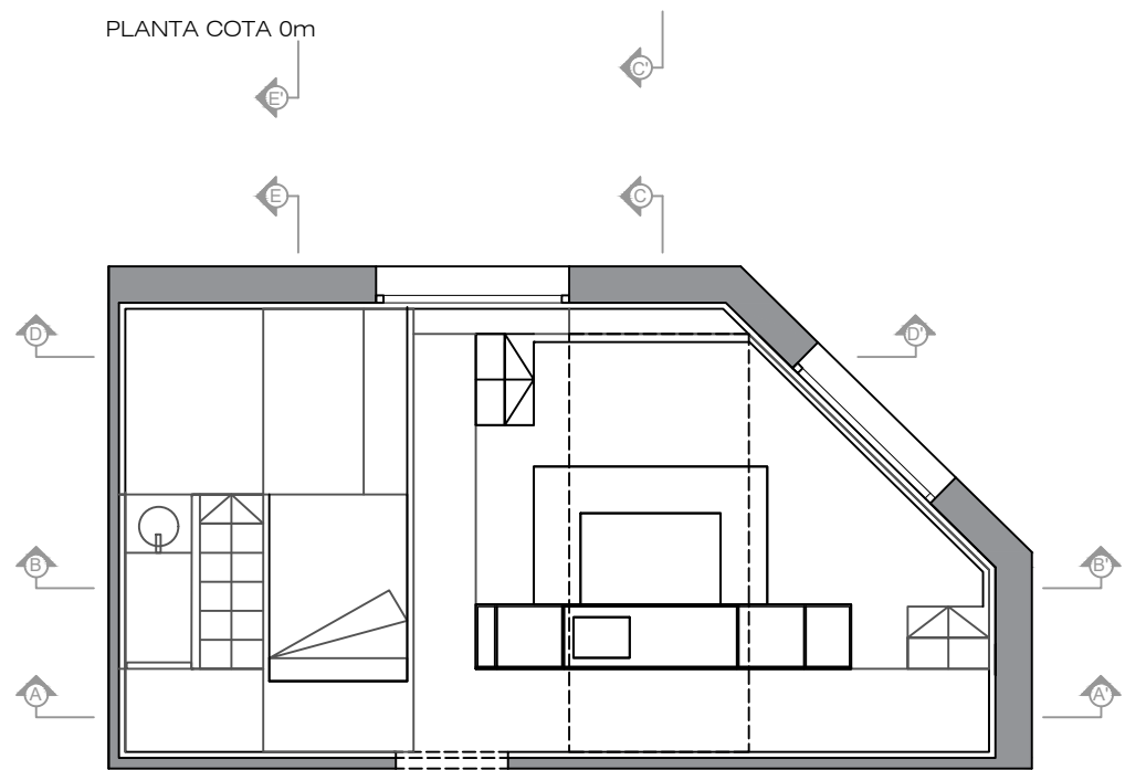
PLANTA COTA 2,10m
