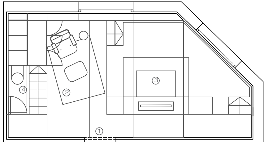
PLANTA COTA 0m
