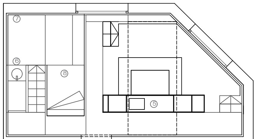
PLANTA COTA 2,10m
