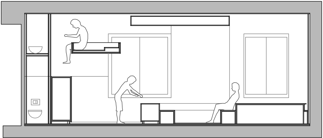
SECCIÓN BB'
