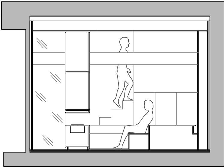
SECCIÓN CC'
