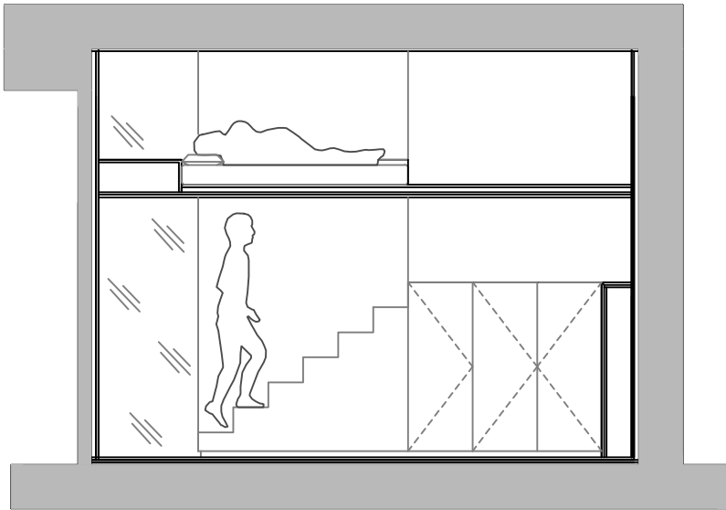
SECCIÓN EE'
